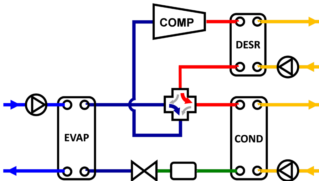
Esquema simplificado de CLASSIC HC con desrecalentador.
