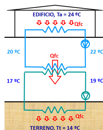
Frío pasivo
