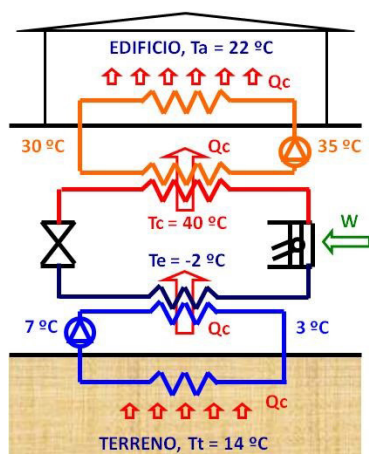
Calefacción
