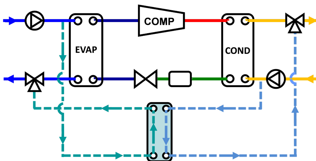
Esquema simplificado del sistema de producción de frío pasivo.
