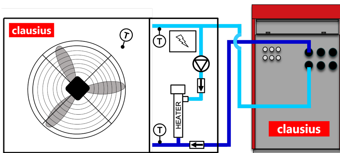
Esquema simplificado, aeroterminia CLAUSIUS
