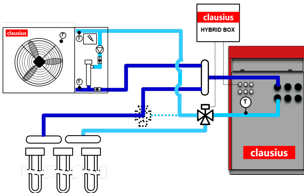
Esquema simplificado, sistema híbrido CLAUSIUS
