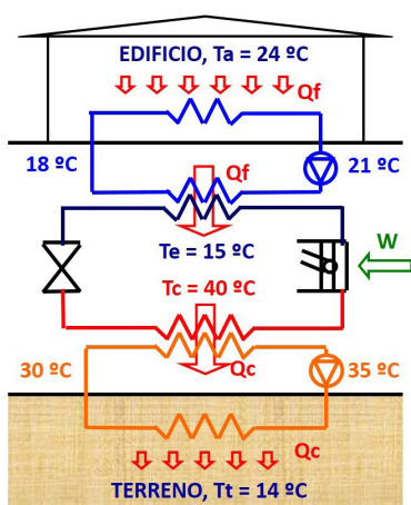
Frío activo
